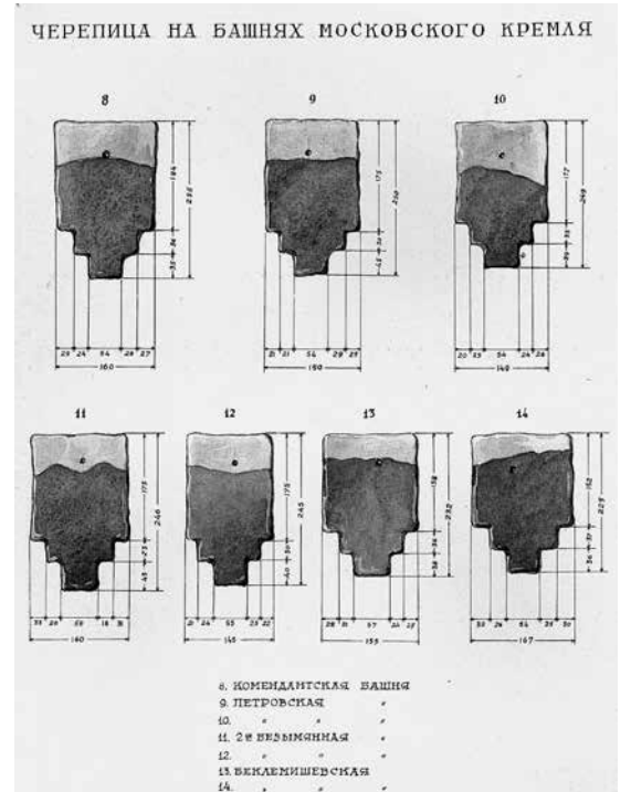
ил.8 Черепица на башняхъ Московскаго Кремля. Таблица с промерами Архив А.В.Филиппова fig.8 Roof tiles on the towers of the Moscow Kremlin. Table with measurements. Archive of A.V.Filippov
