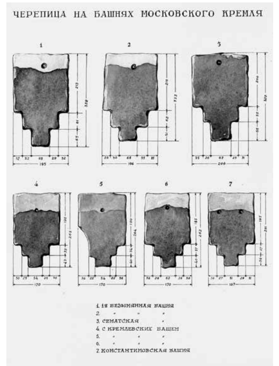
ил.5 Анкета с описаніем (а) и зарисовкой черепицы кремлевскихъ башен (б) из коллекціи артели художниковъ гончаровъ «Мурава». Составлена 22.07.1913. Архив А.В.Филиппова fig.5 Questionnaire with description (a) and sketch of the tiles of the Kremlin towers (б) from the collection of the potters' artel "Murava". Compiled on 22.07.1913 Archive of A.V.Filippov
