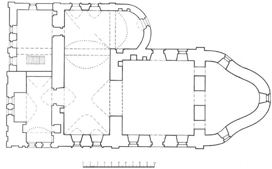
ил. 5 Схема плана Троицкого собора, выполненная на основании обмера 1985 г. и генплана монастыря 1926 г.
